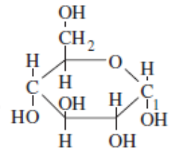
\alpha -Glucopyranose
