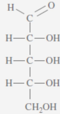
Ribose
