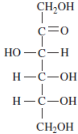
Fructose
