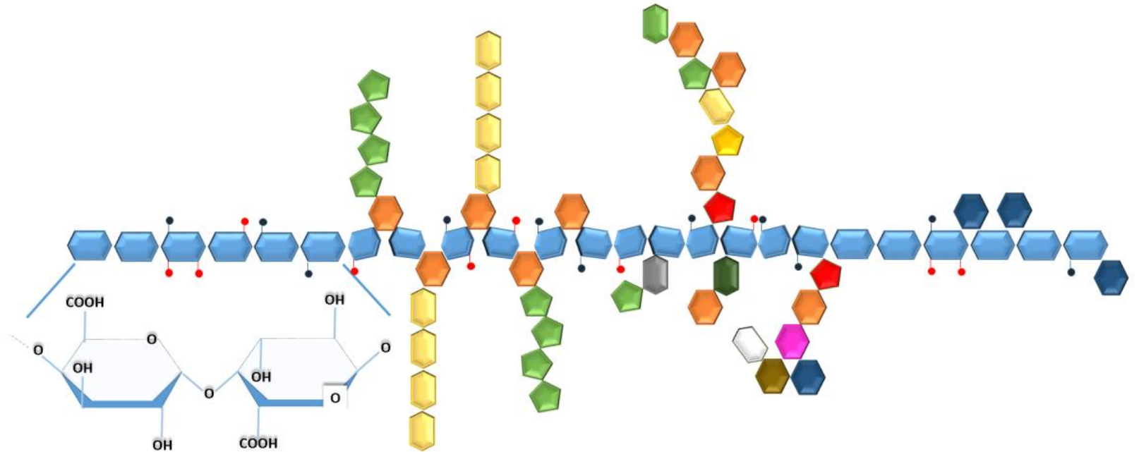
HOMOGALACTURONAN
