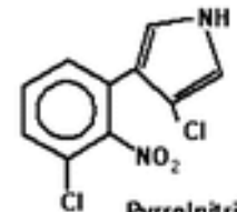
Pyrrolnitrin
