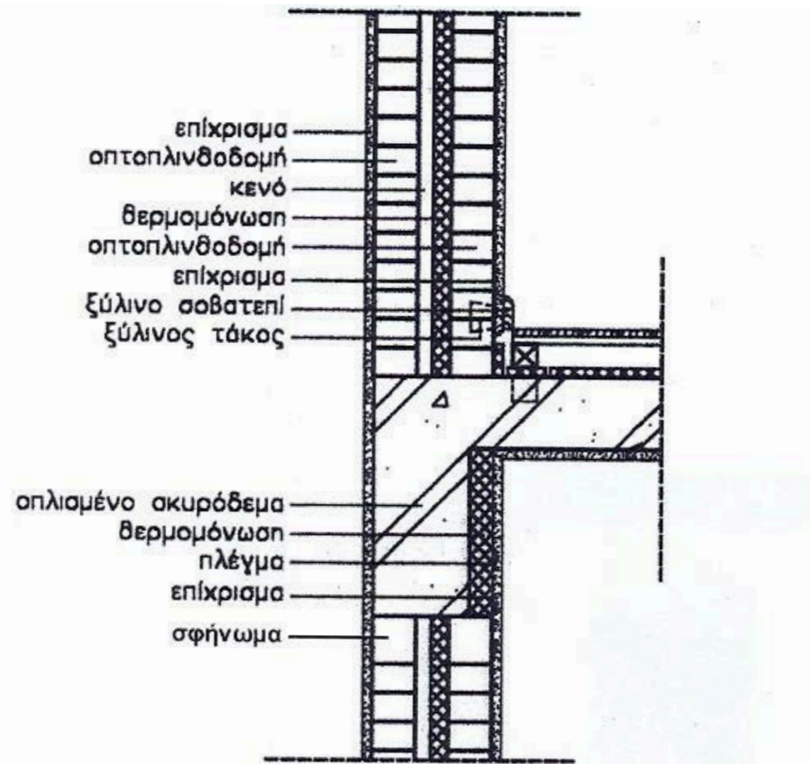
ΛΕΠΤΟΜΕΡΕΙΑ ΤΟΙΧΟΠΟΙΙΑΣ
