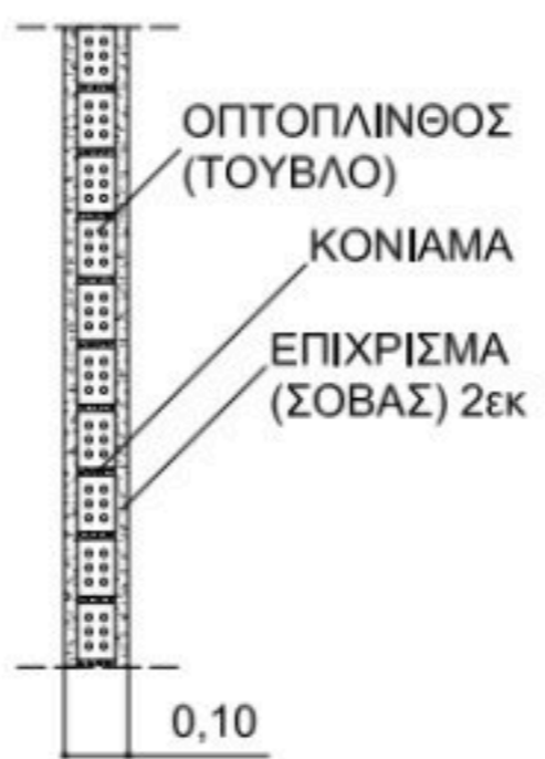
ΤΟΜΗ ΜΠΑΤΙΚΗΣ ΟΠΤΟΠΛΙΘΟΔΟΜΗΣ ΜΕ ΣΥΡΟΜΕΝΟ ΣΥΣΤΗΜΑ
