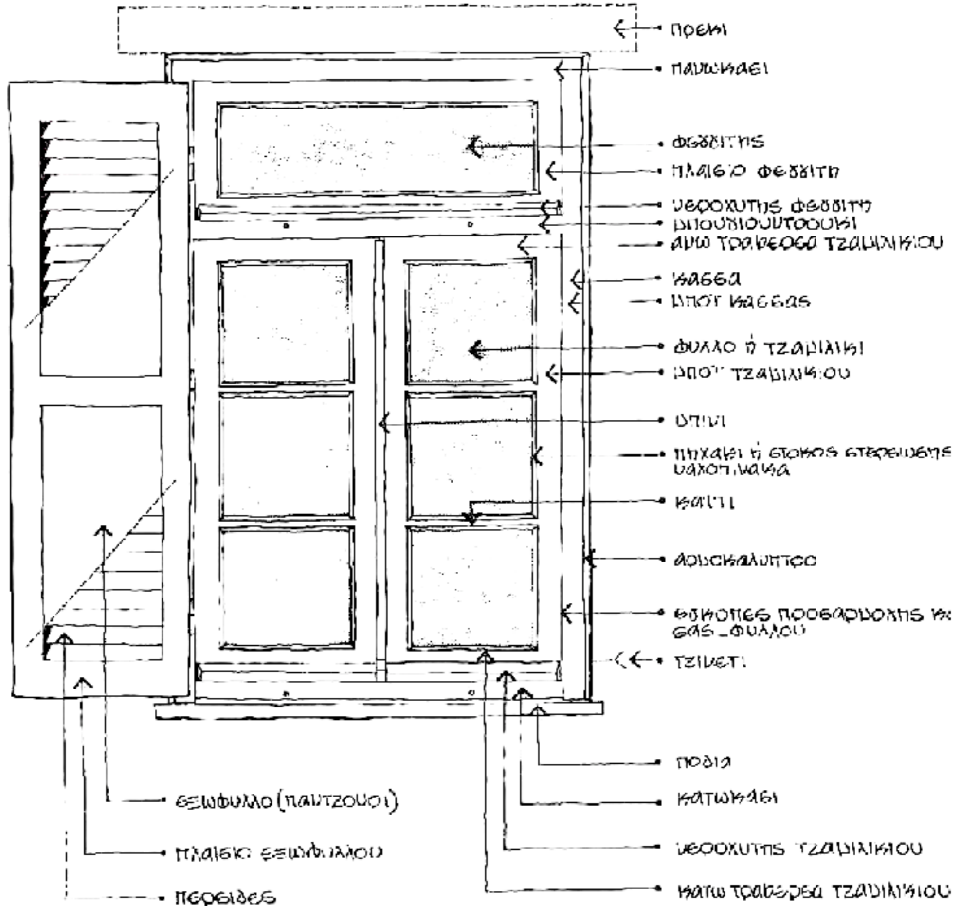
ΕΞΩΤΕΡΙΚΗ ΟΥΤΗ ΕΥΛΙΝΟΥ ΠΑΡΑΘΕΡΟΥ
