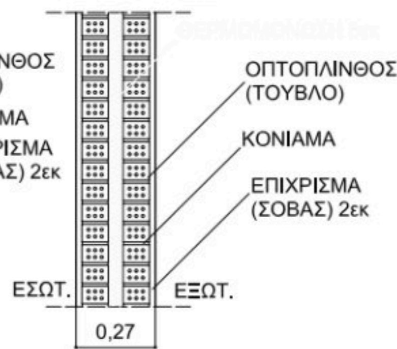
ΤΟΜΗ ΜΠΑΤΙΚΗΣ ΟΠΤΟΠΛΙΘΟΔΟΜΗΣ ΜΕ ΘΕΡΜΟΝΩΣΗ
