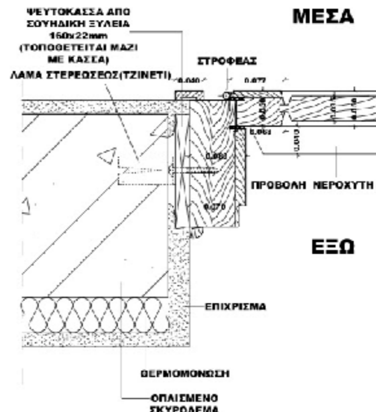
ΛΕΠΤΟΜΕΡΕΙΕΣ ΚΑΤΩΨΗΣ
