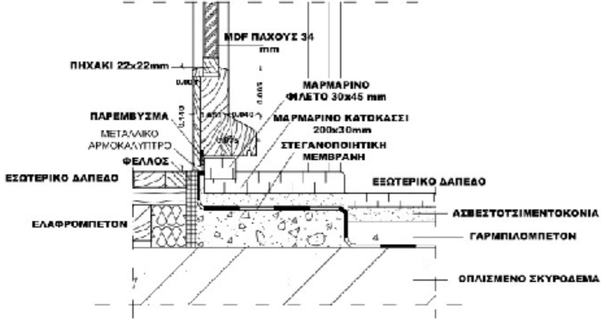
ΛΕΠΤΟΜΕΡΕΙΕΣ ΤΟΜΗΣ
