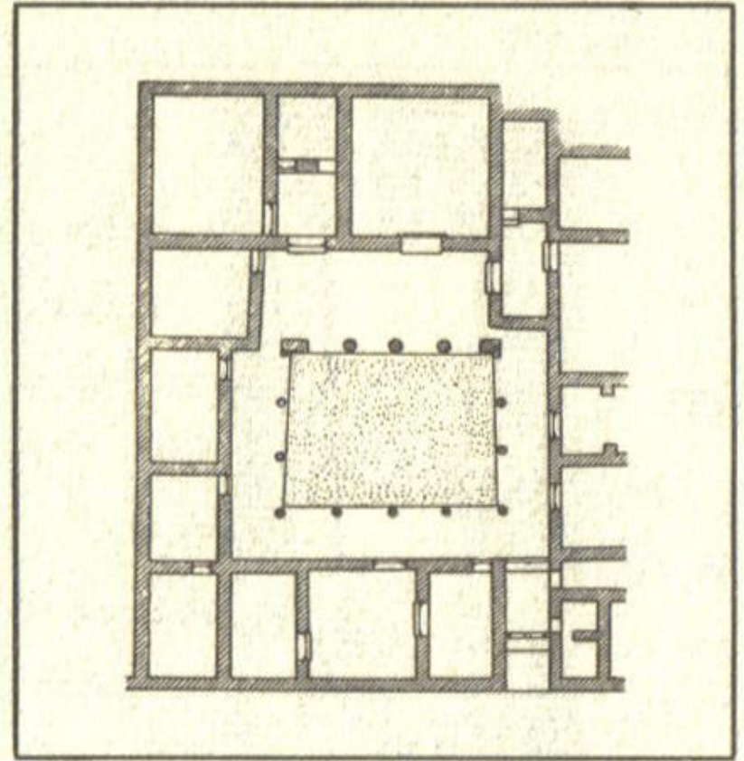
Πριήνη. Σπίτι με εσωτερική αυλή και περιστύλιο.
