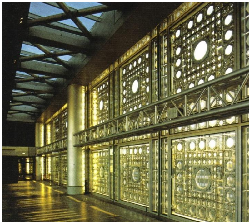
Nouvel J., Institut du Monde Arabe (1981-87), άποψη του ηλεκτρονικού συστήματος ηλιοπροστασίας, από το εσωτερικό του κτιρίου.
