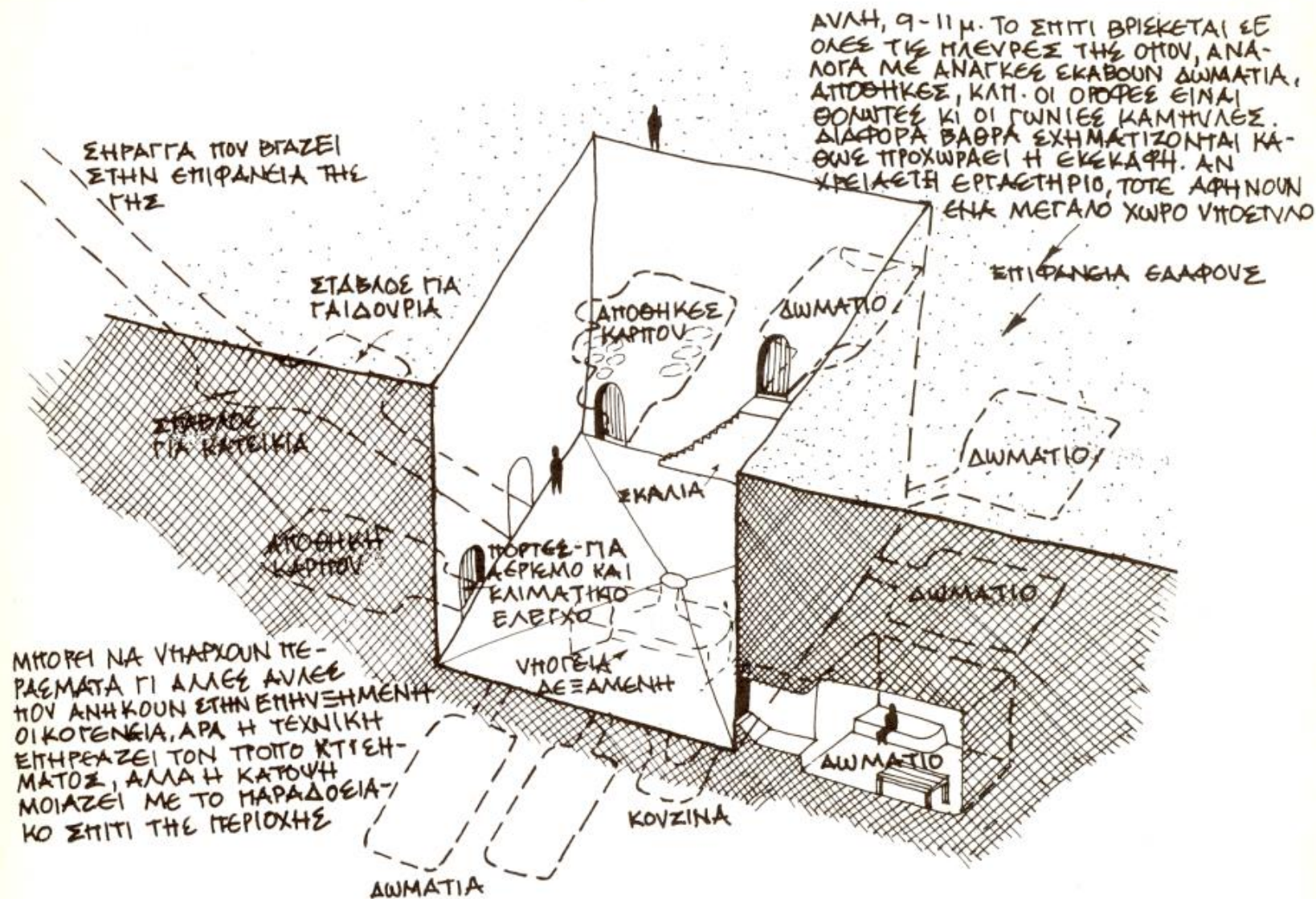
Άξονομετρική τομή κατοικίας τῶν Matmata στὴ Σαχάρα
