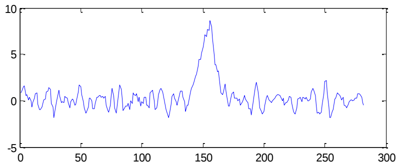
Συνέλιξη με [1, 1, 1, 1, 0, -1, -1, -1, -1]
