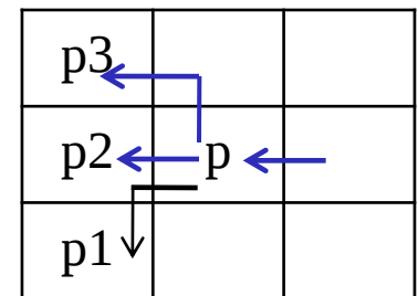
Κατεύθυνση K=4
