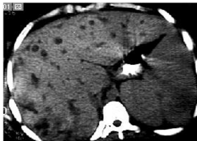
Μετασχηματισμένη εικόνα
