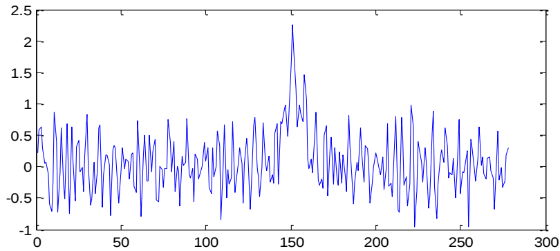
Συνέλιξη με [1, 0, -1]
