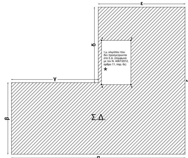
σχεδιάγραμμα ισογείου
